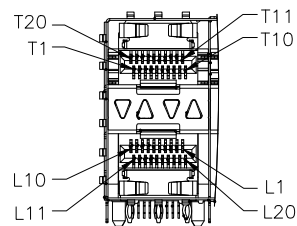
DETAIL A 1:1
