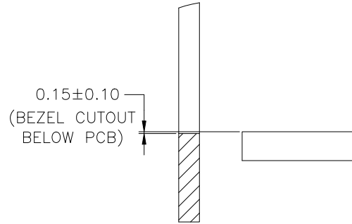
DETAIL K 2:1
