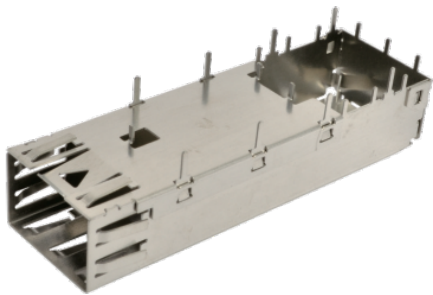
SFP 1X1 Cage
