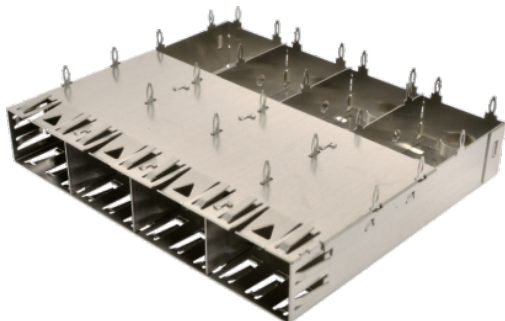
SFP 1X4 Cage
